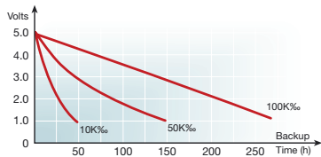
Figure 27. 5.6F - LJ Series
