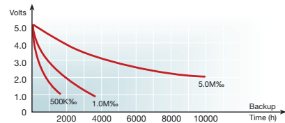
Figure 28. 5.6F - LJ Series
